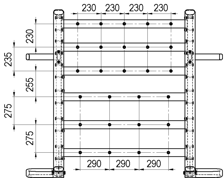
视图 A
